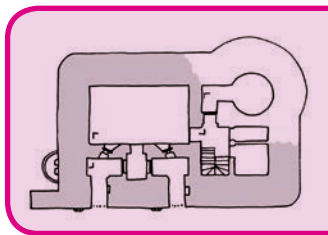
Schemat schronu typu Regelbau 105C, rys. RS
